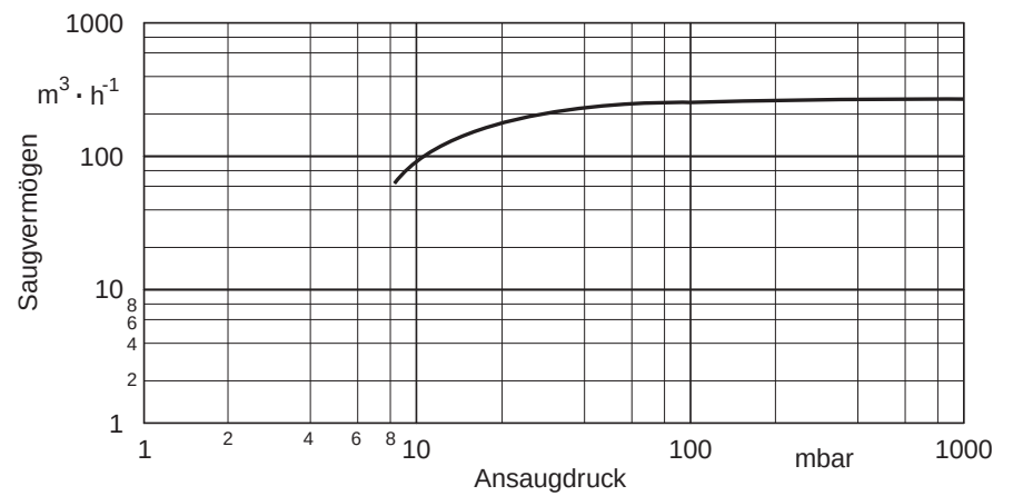
Abb. 2.39 Saugvermögenskurve einer ALL-ex 250
