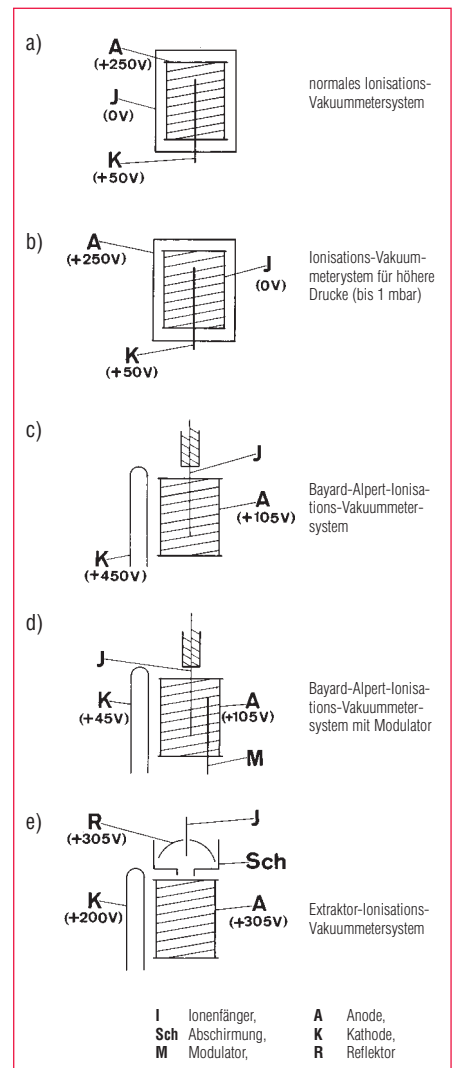
Abb. 3.16 Schematische Darstellung des Elektrodenaufbaues verschiedener Ionisations-Vakuummeter-Meßsysteme
