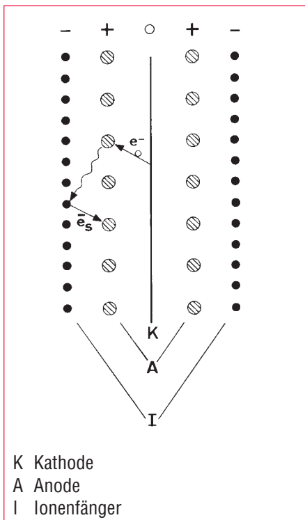
Abb. 3.15 Zur Erklärung des Röntgeneffektes in einer normalen Ionisations-Vakuummeter-Ende. Die von der Kathode K emittierten Elektronen e^- prallen auf die Anode A und lösen dort eine weiche Röntgenstrahlung (Photonen) aus. Diese trifft zum Teil auf den Ionenfänger I und erzeugt dort Photoelektronen aus e^- .
