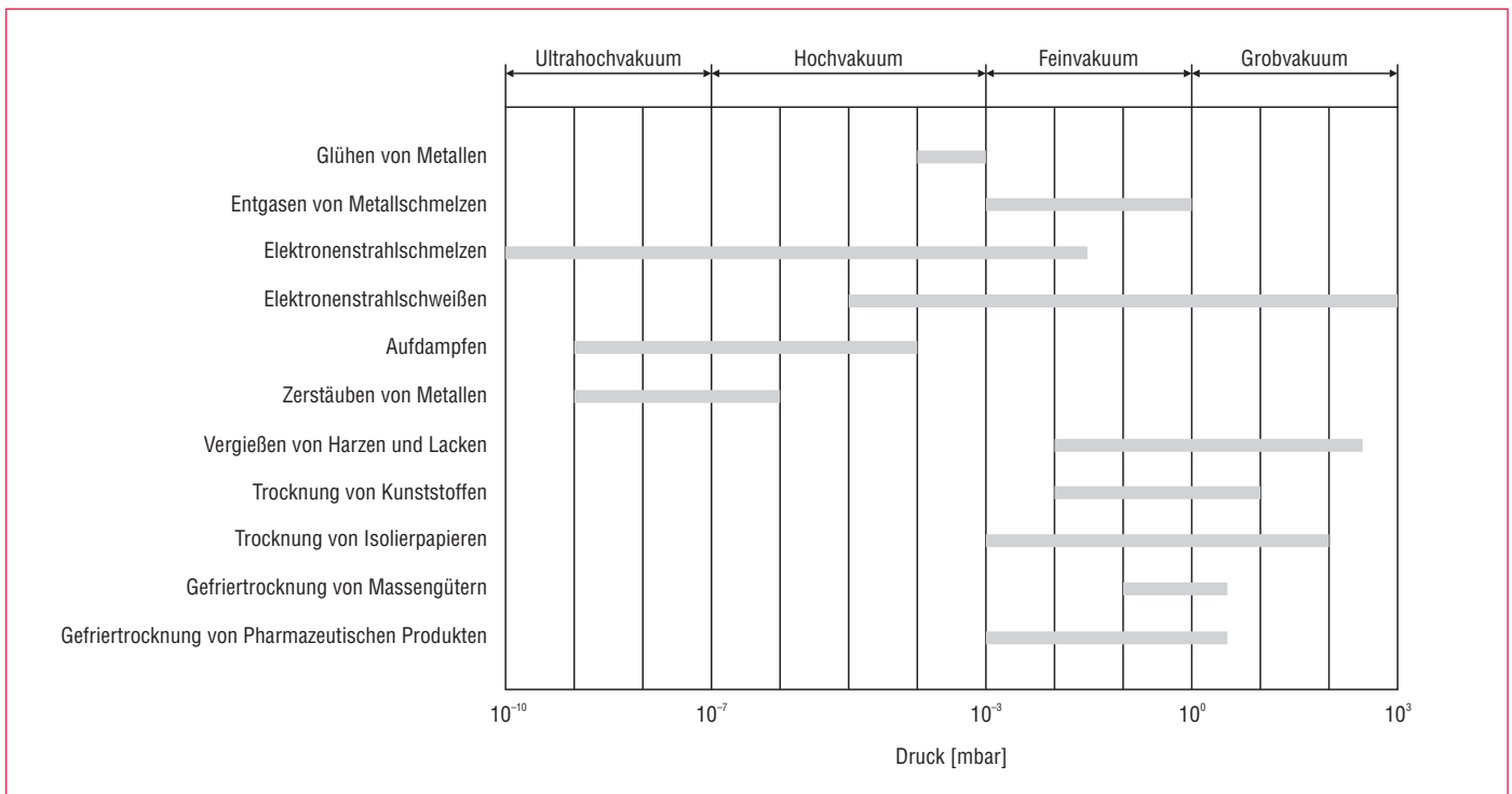
Abb. 7.1 Druckgebiete in denen verschiedenen Vakuumverfahren arbeiten
