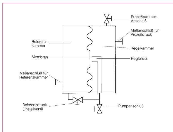
Abb. 3.27 Prinzip des Membranreglers
