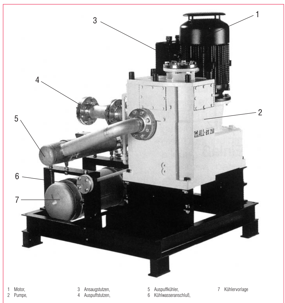
Abb. 2.36 »ALL-ex«-Pumpe
