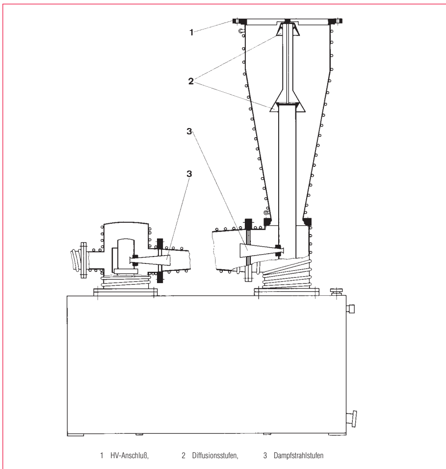
Abb. 2.47 Schema einer Öldampfstrahl-(Booster-)Pumpe
