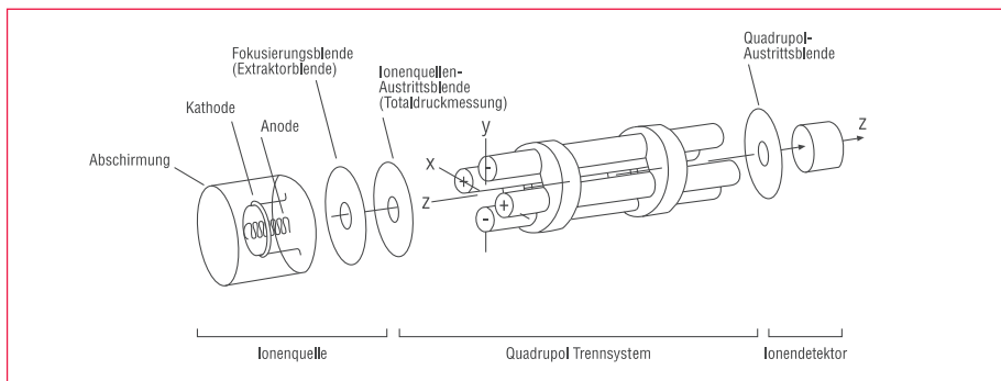
Abb. 4.2 Schema Quadrupol-Massenspektrometer
