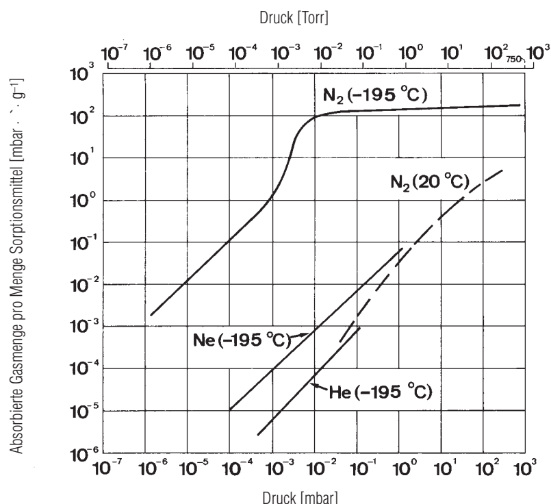
Abb. 2.60 Adsorptionsisothermen von Zeolith 13X für Stickstoff bei -195^\circ\text{C} und 20^\circ\text{C} , sowie für Helium und Neon bei -195^\circ\text{C}
