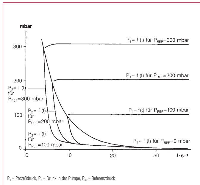
Abb. 3.28 Regelverhalten eines Membranreglers
