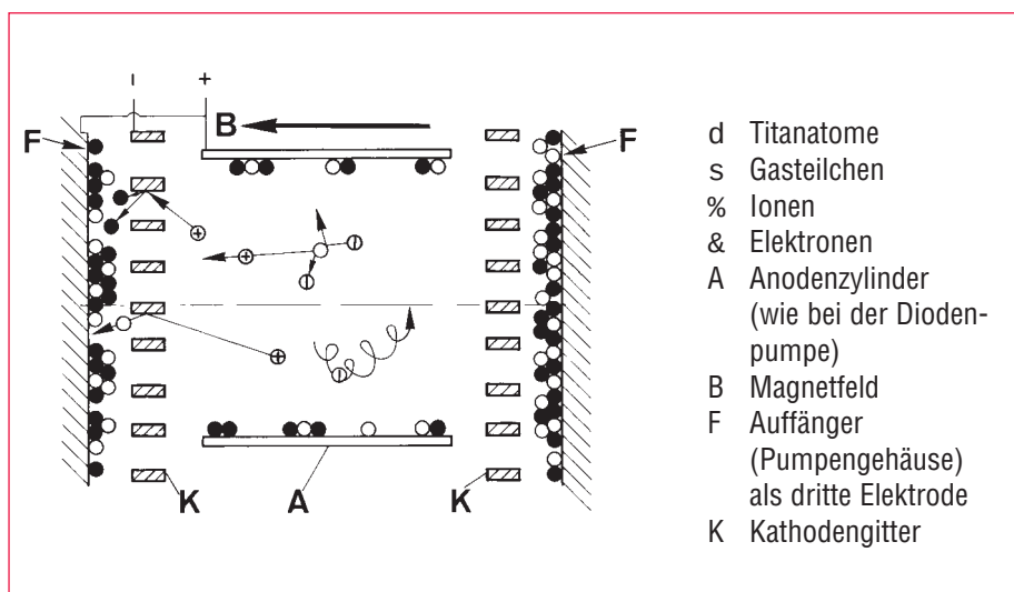
Abb. 2.63 Elektrodenkonfiguration einer Trioden-Ionenzerstäuberpumpe
