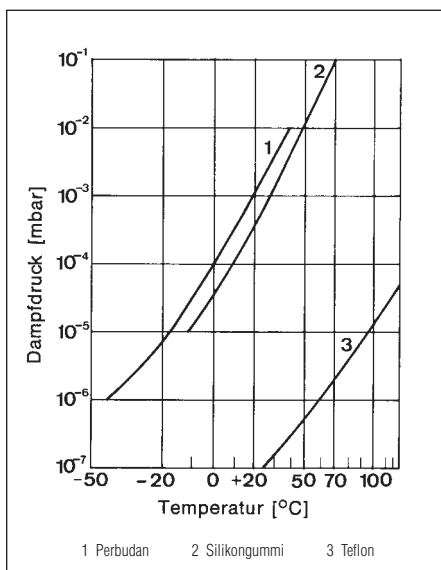
Abb. 9.14: Dampfdruck von nichtmetallischen Dichtungsmitteln (die Dampfdruckkurve für Viton liegt zwischen den Kurven für Silikongummi und Teflon).
