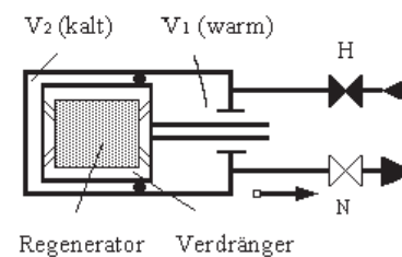
Abb. 2.66 Phasen der Kälteerzeugung mit einem einstufigen Kaltkopf nach dem Gifford-McMahon Prozeß
