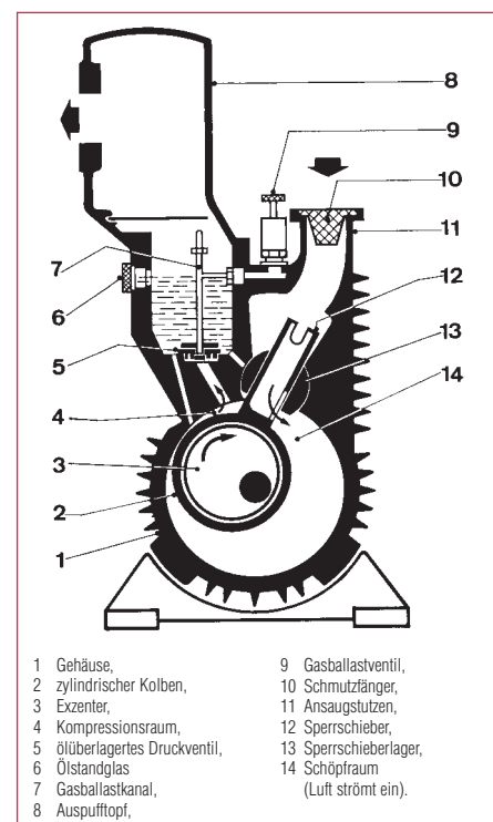
Abb. 2.9 Schnitt durch eine einstufige Sperrschieberpumpe (Einblockbauart).
