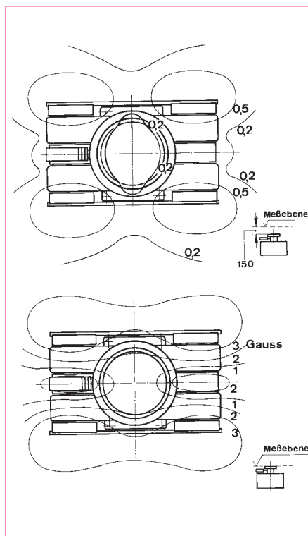
Abb. 2.64 Strommagnetfeld einer Ionen-Zerstäuberpumpe in 2 Ebenen parallel zur Fläche des Ansaugflansches (siehe Teilbilder). Kurven gleichen Betrages der magnetischen Induktion B in Gauß. 1 Gauß = 1 \cdot 10^{-4} Tesla
