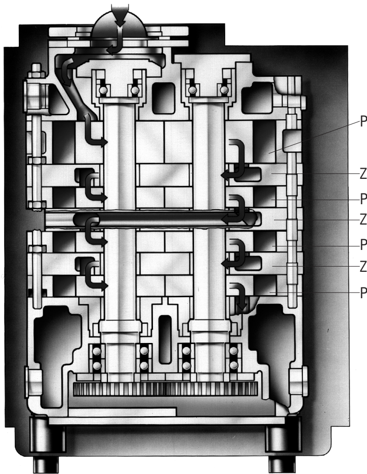
Abb. 2.24 Anordnung der Stufen und Führung des Gasstroms. P = Pumpstufe Z = Zwischenring
