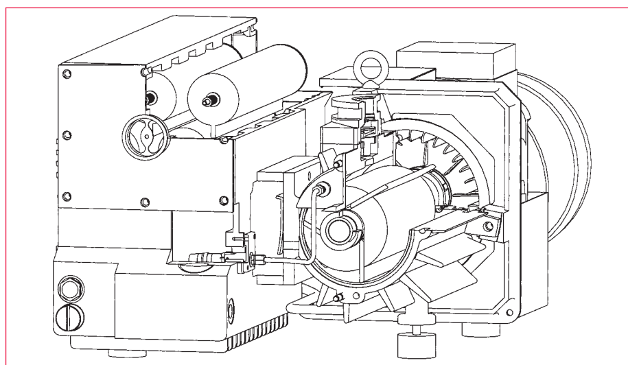
Abb. 2.8b SOGEVAC Pumpe SV 300 mit drei tangentialen Schiebern
