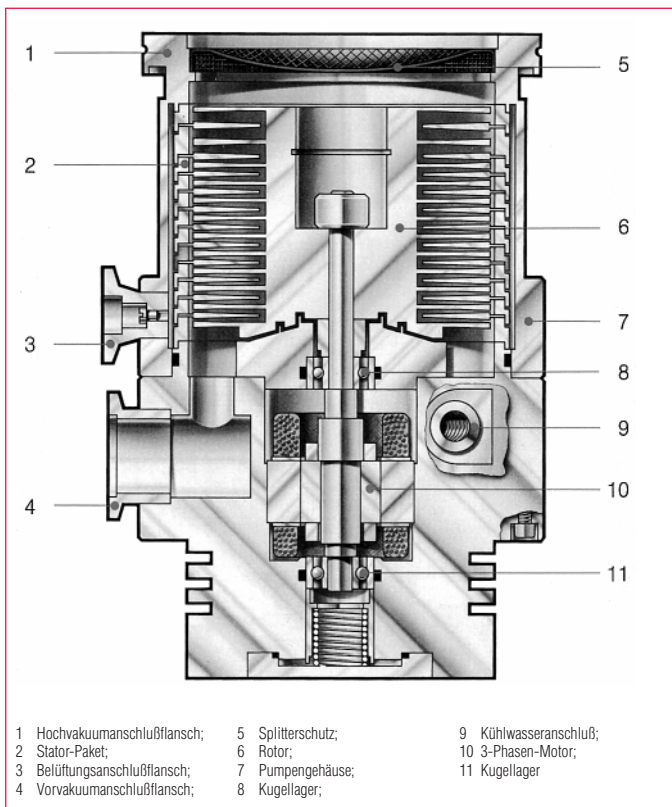
Abb. 2.52 Prinzipische Zeichnung der fettgeschmierten Turbo-Molekularpumpe TURBOVAC 151
