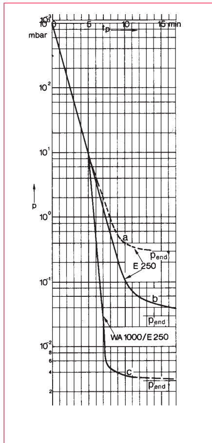
Abb. 2.77 Abspumpzeit t_p eines 5 m 3 Behälters mit einer Sperrschieberpumpe E 250 mit einem Nennsaugvermögen von 250 m 3 /h mit (a) und ohne Gasballast (b), sowie der Wälzkolben-/Sperrschieber-Pumpenkombination WA1001/E250 für einen Einschaltzeitpunkt der WA 1001 von 10 mbar (c).
