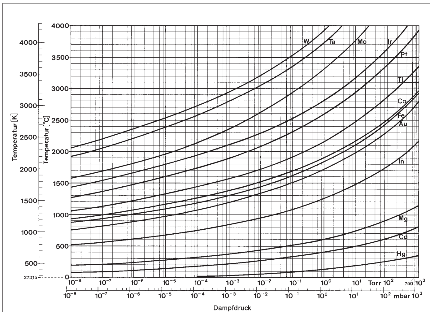
Abb. 9.13: Sättigungsdampfdruck vakuumtechnisch wichtiger Metalle
