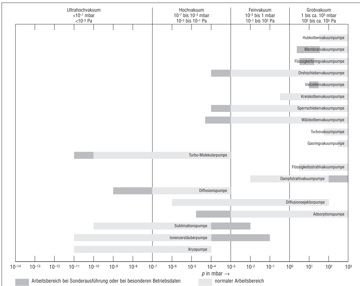
Abb. 9.16: Gebräuchliche Arbeitsbereiche von Vakuumpumpen
