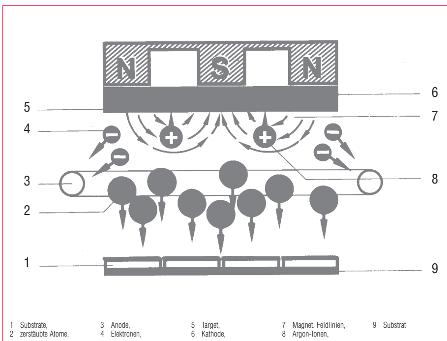
Abb. 7.3 Funktionschema einer Hochleistungs-Kathodenzerstäubungsanordnung
