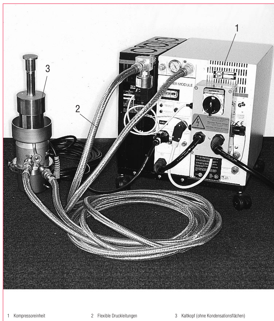
Abb. 2.65 Gesamtaufbau einer Refrigerator-Kryopumpe
