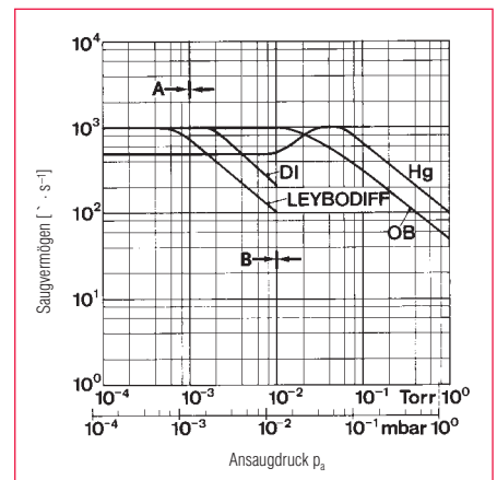
Abb. 2.48 Saugvermögen verschiedener Treibmittelpumpen in Abhängigkeit vom Ansaugdruck bezogen auf Nennsaugvermögen von 1000 \text{ l} \cdot \text{s}^{-1} . Ende des Arbeitsbereiches von Öldampfstrahlpumpen (A) und von Öldiffusionspumpen (B)
