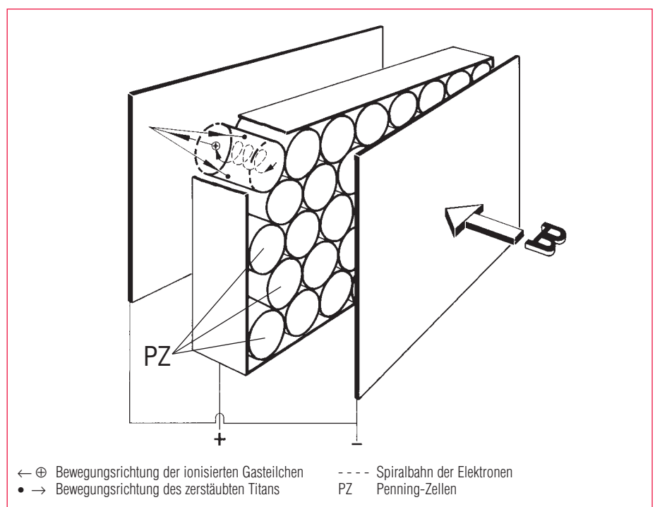
Abb. 2.61 Zur Wirkungsweise der Ionen-Zerstäuberpumpe
