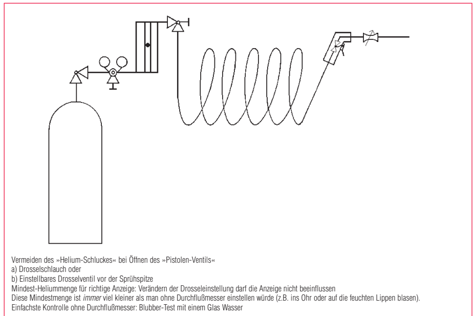
Abb. 5.15 Heliumsprüheinrichtung
