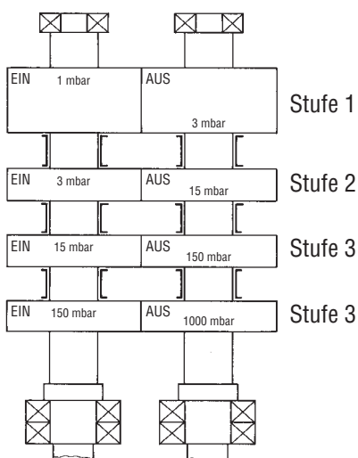
Abb. 2.25 Druckverhältnisse in den Pumpstufen 1 bis 4
