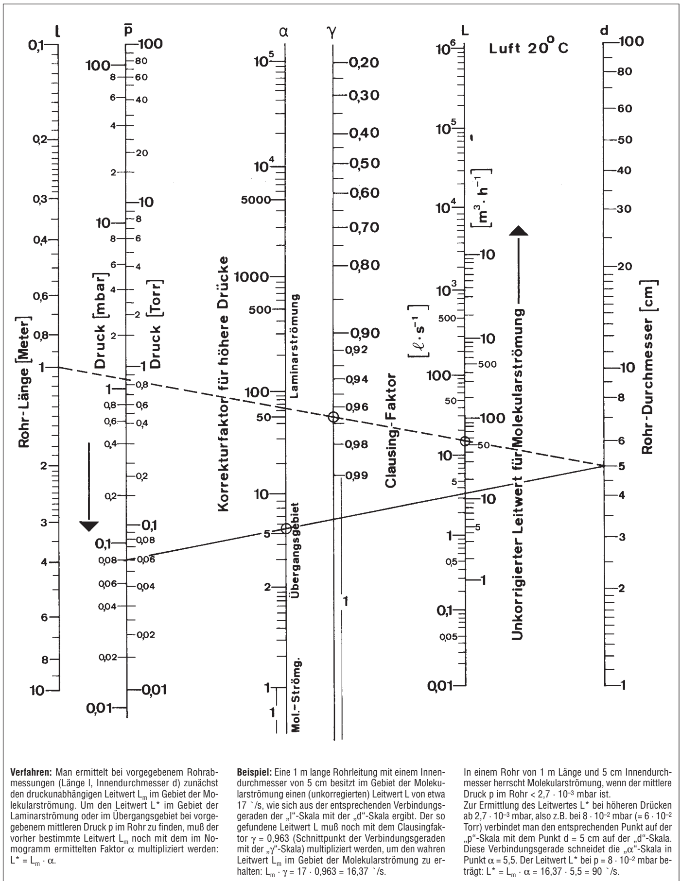
Abb. 9.9: Nomogramm zur Ermittlung der Leitwerte von Rohrleitungen (Luft, 20°C) im gesamten Druckgebiet.
