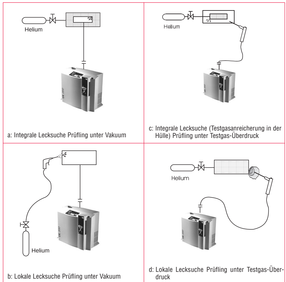
Abb. 5.4 Lecksuchmethoden – Fachausdrücke
