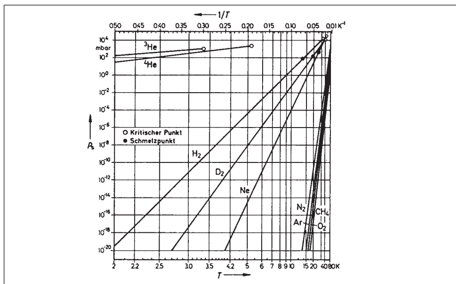
Abb. 9.15: Sättigungsdampfdrücke p_s verschiedener kryotechnisch wichtiger Stoffe im Temperaturbereich T = 2 \dots 80 K.
