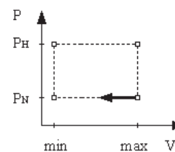
Abb. 2.66 Phasen der Kälteerzeugung mit einem einstufigen Kaltkopf nach dem Gifford-McMahon Prozeß
