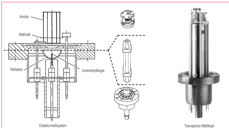
Abb. 4.3 Quadrupol-Massenspektrometer – Extraktor-Ionisations-Vakuummeter
