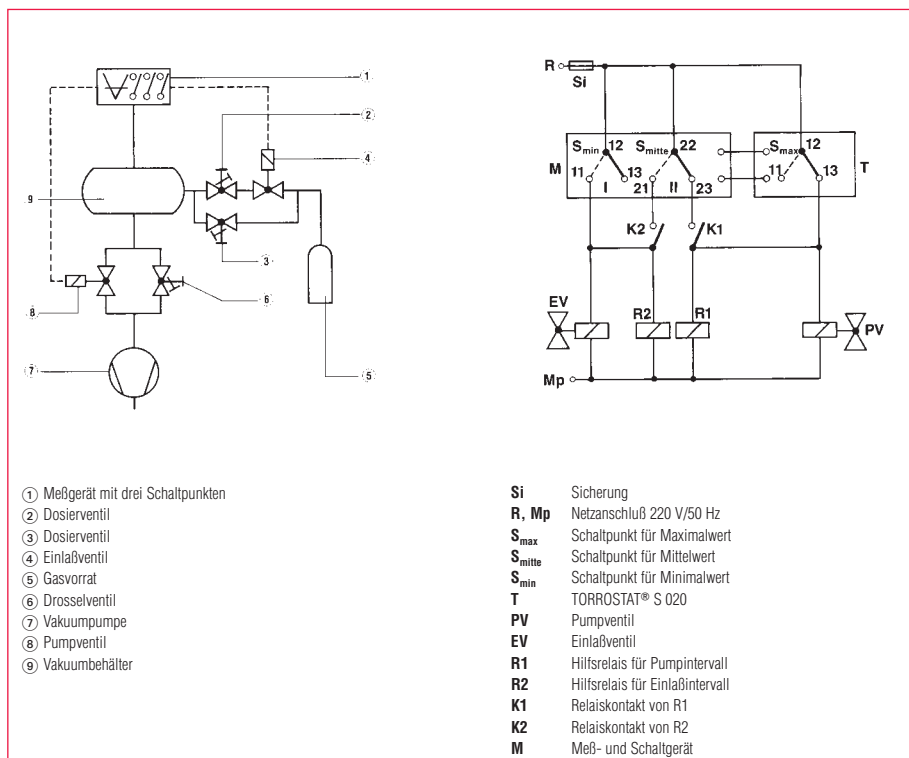
Abb. 3.24 Dreipunktregelung
