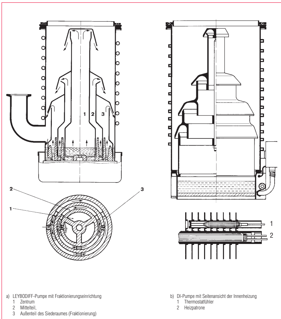
Abb. 2.45 Schematische Darstellung der wesentlichen Unterschiede bei Öldiffusions-Pumpen von Leybold
