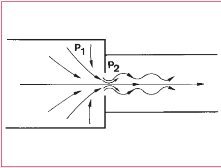
Abb. 1.2 Strömung eines Gases durch eine Öffnung (A) bei hohen Drücken (viskoser Strömung)
