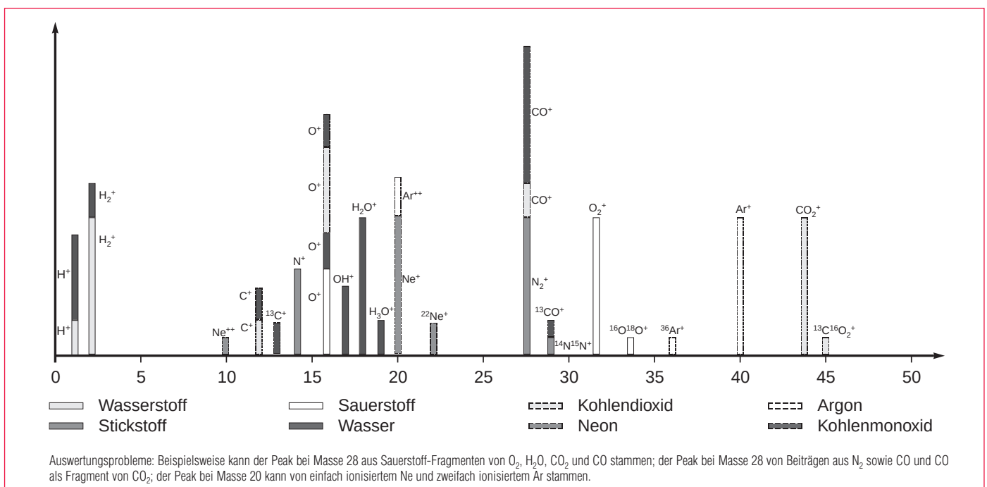
Abb. 4.15 Modellspektrum
