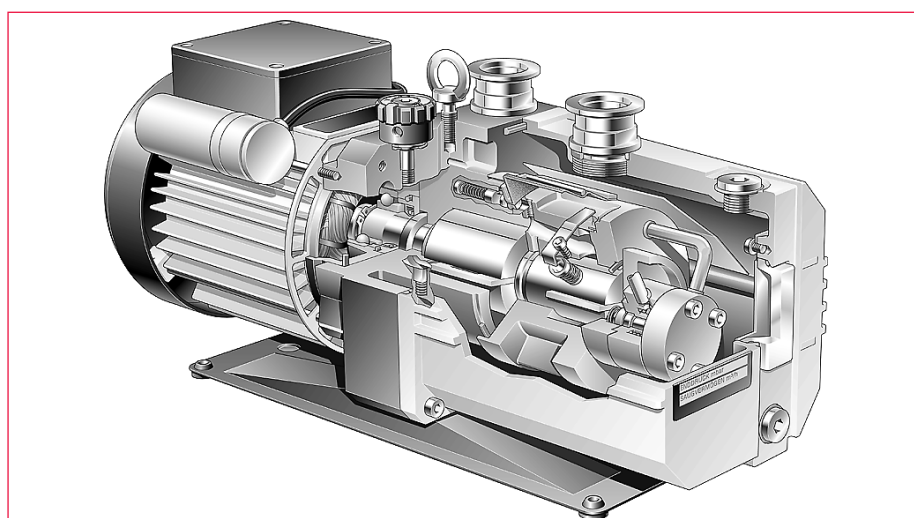
Abb. 2.8a Schnitt durch eine zweistufige Drehschieberpumpe (TRIVAC E)
