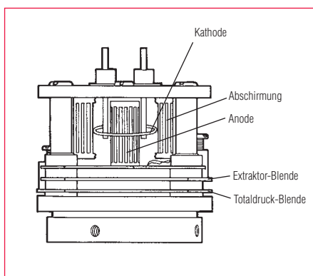
Abb. 4.4 Offene Ionenquelle
