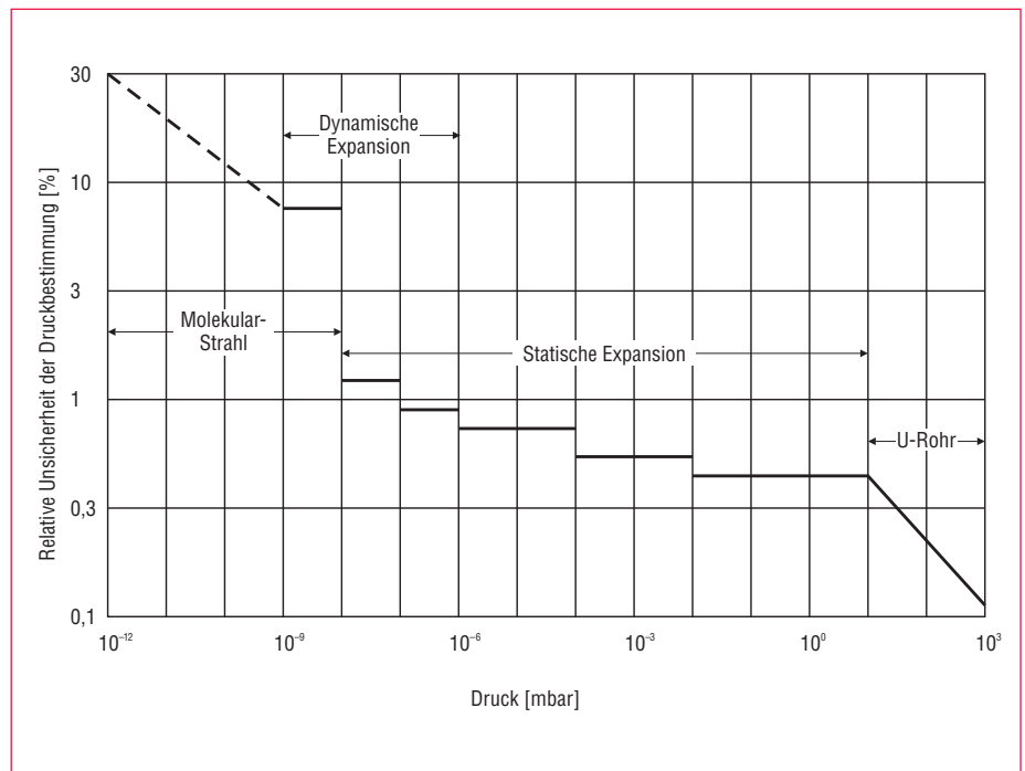
Abb. 3.17 Druckskala der Physikalisch-Technischen Bundesanstalt (PTB), Berlin, (Stand August 1984) für Edelgase, Stickstoff und Methan
