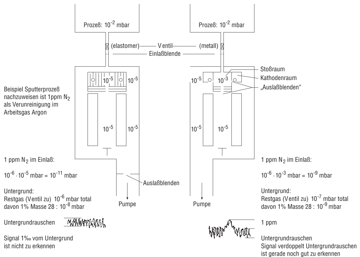
Abb. 4.8 Offene Ionenquelle (links) und geschlossene Ionenquelle (rechts)
