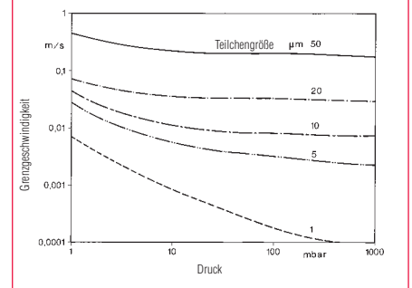
Abb. 2.31 Sinkgeschwindigkeit in Abhängigkeit vom Druck p . Parameter: Teilchengröße
