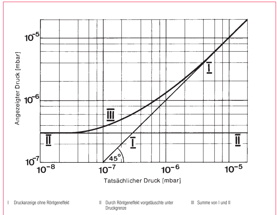
Abb. 3.14 Durch den Röntgeneffekt bei einer normalen Ionisations-Vakuummeterröhre vorgetäuschte untere Druckmeßgrenze.
