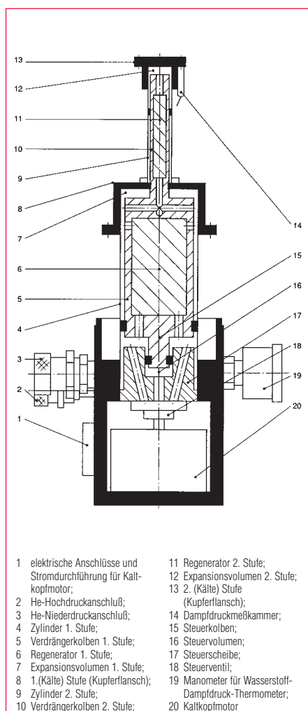
Abb. 2.67 zweistufiger Kaltkopf
