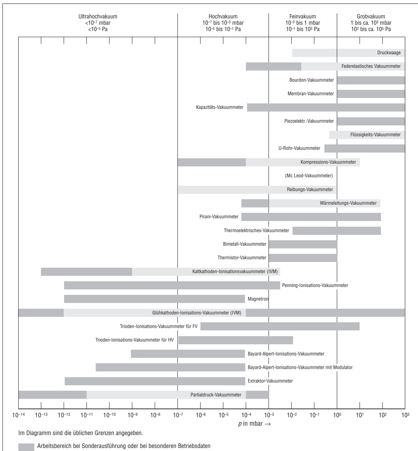
Abb. 9.16a: Meßbereiche gebräuchlicher Vakuummeter (VM) nach DIN 28400, Teil 3, 1992
