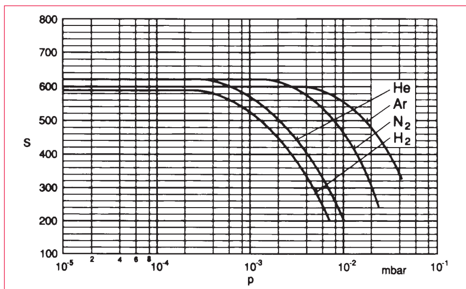
Abb. 2.54 Saugvermögenskurven einer TURBOVAC 600 für H_2 , He, N_2 und Ar
