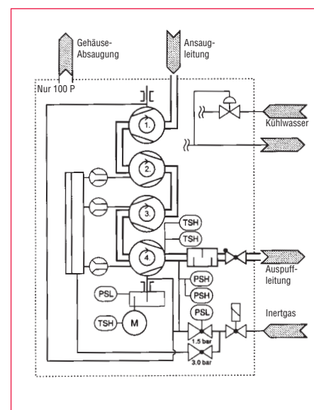
Abb. 2.29b Funktionsschema der DRYVAC P
