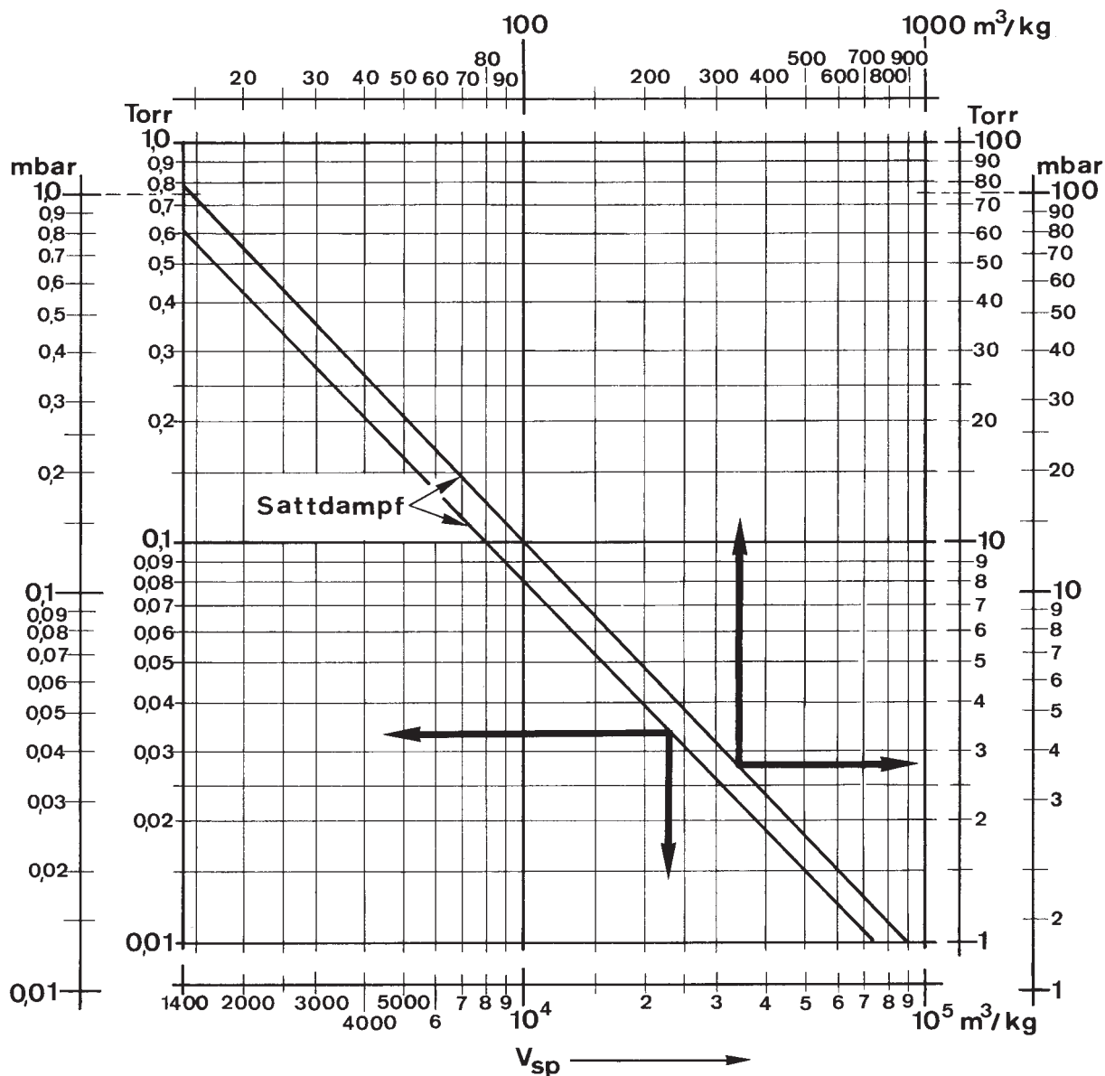
Abb. 9.17: Spezifischer Rauminhalt V_{sp} von Wasserdampf in m^3/kg bei 0,013 bis 133 mbar (Satttdampf).
