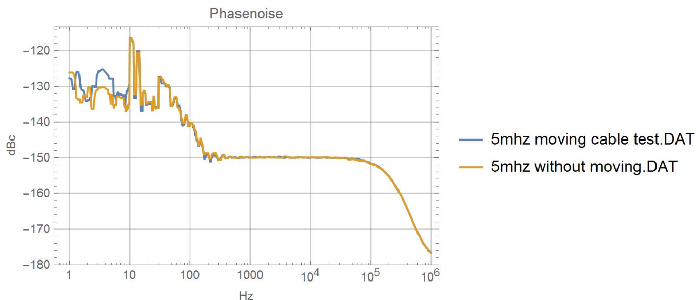
5mhz_moving_cable_test.pdf
